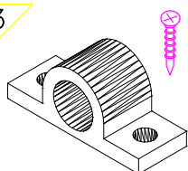
Prowadnik pręta baszkiowego Wkręt \emptyset 3 \times 16 S
