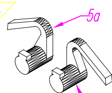
Haczyk górny i dolny zamka baszkiowego
